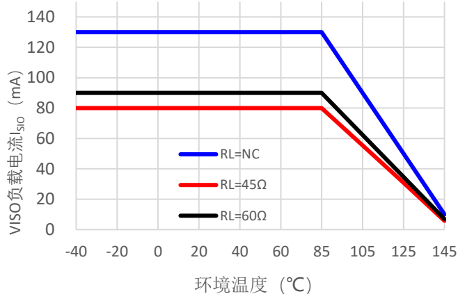
图 7.9-12 V_{ISO} 最大负载可用电流 I_{ISO} 随器件环境温度的变化 CANH 和 CANL 之间 R_L 接不同电阻 DR = 1Mbps, CANH 和 CANL 之间 C_L = 2nF
