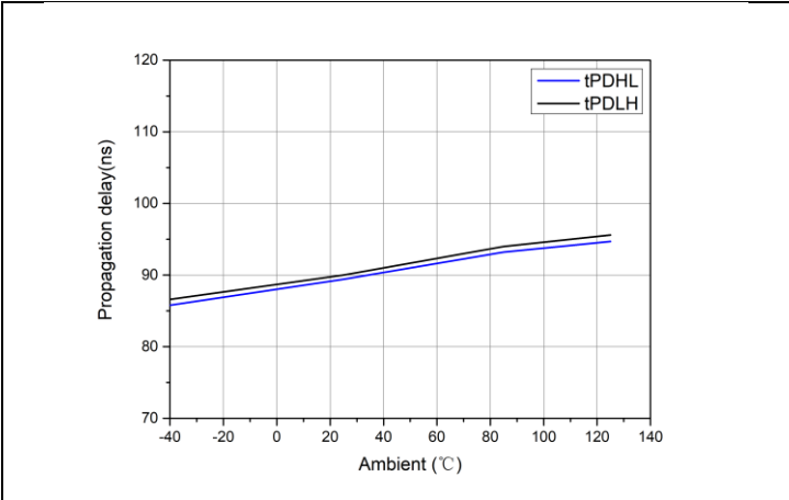
图 7-7 传输延时与温度关系
