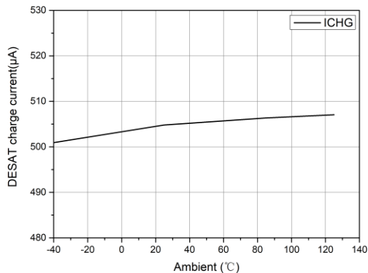
图 7-13 DESAT 充电电流( I_{CHG} )与温度关系
