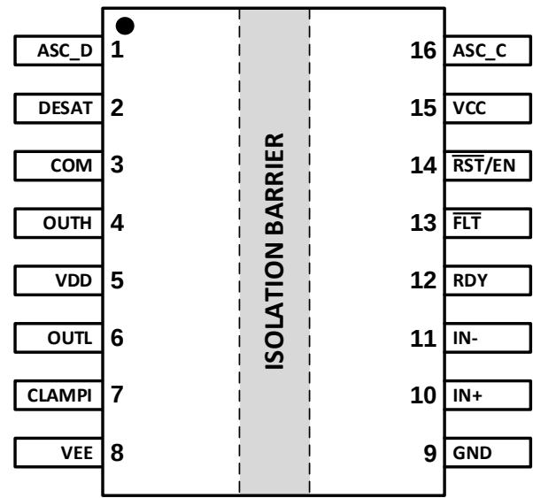
图 6-1 CA-IS321xNNW-Q1/ CA-IS321xSNW-Q1 引脚配置
