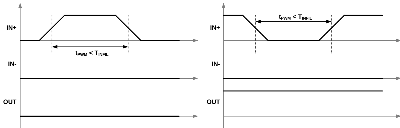
图 8-3 IN+ ON/OFF 滤波器
