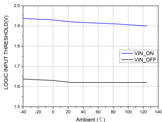
图 7-5 逻辑输入阈值与温度的关系
