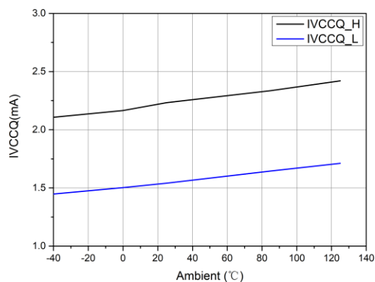
图 7-1 VCC 静态工作电流与温度关系
