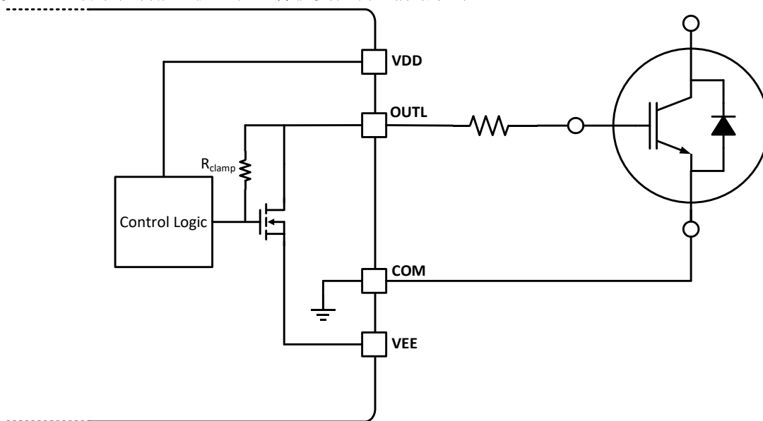
图 9-4 主动下拉
