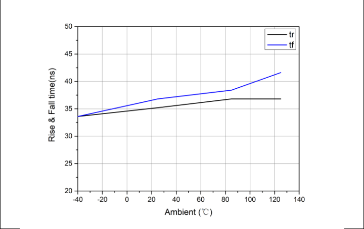
图 7-10 上升&下降时间与温度的关系 (CL=10nF)
