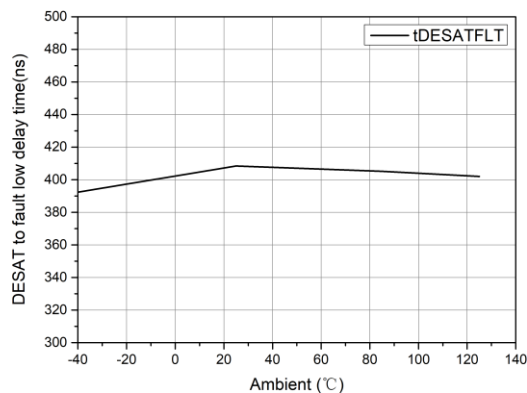
图 7-18 DESAT to Fault 延时( t_{DESATFLT} )与温度关系
