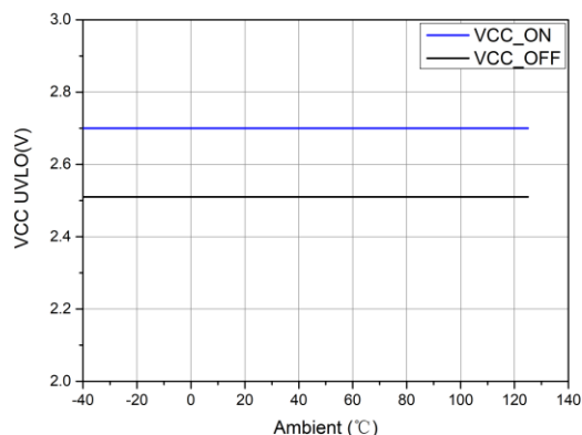
图 7-3 VCC UVLO 与温度的关系
