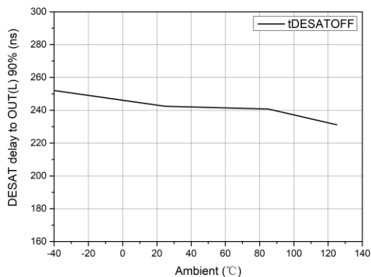
图 7-17 DESAT 关断延时( t_{DESATOFF} )与温度关系
