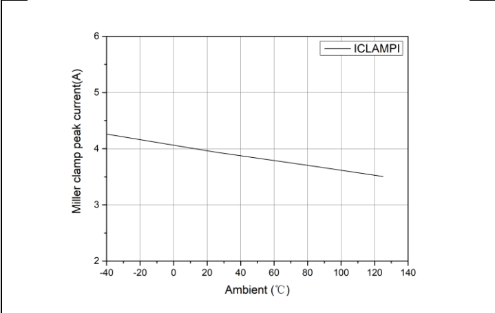
图 7-11 米勒钳位峰值电流与温度的关系
