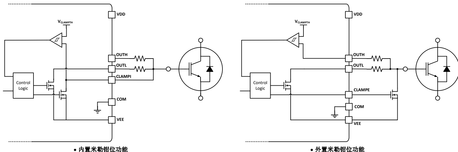
图 9-6 有源米勒钳位
