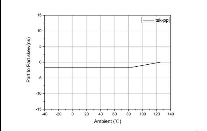
图 7-9 延时匹配与温度的关系
