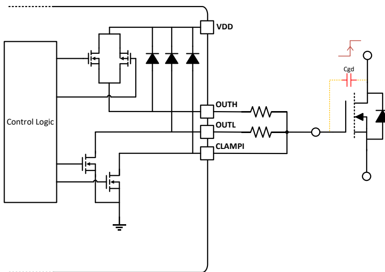
图 9-5 短路钳位
