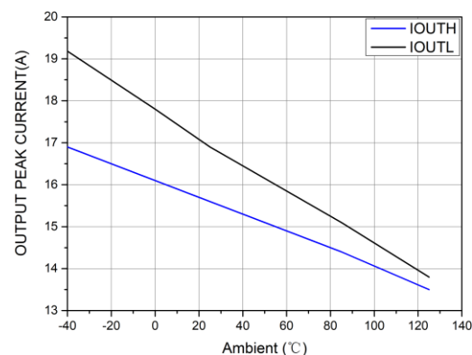
图 7-6 输出峰值电流与温度的关系 (C L =180nF)
