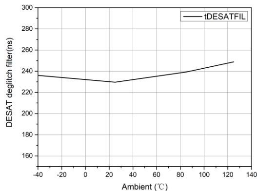
图 7-16 DESAT 滤波时间( t_{DESATFIL} )与温度关系
