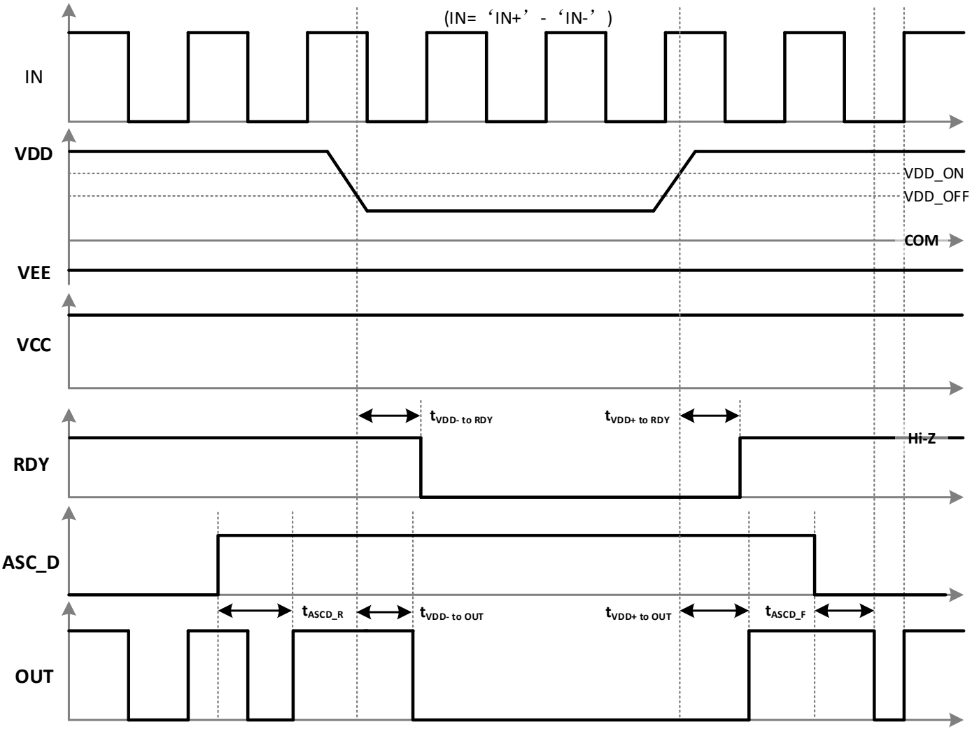
图 8- 14 VDD UVLO 时 ASC_D 保护时序
