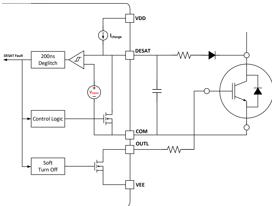
图 9-8 软关断
