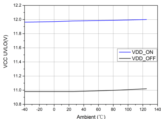
图 7-4 VDD UVLO 与温度的关系
