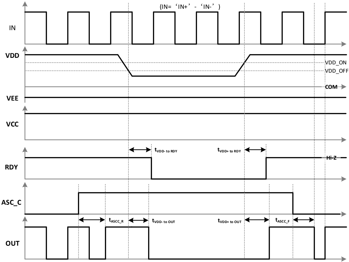
图 8- 12 VDD UVLO 时 ASC_C 保护时序
