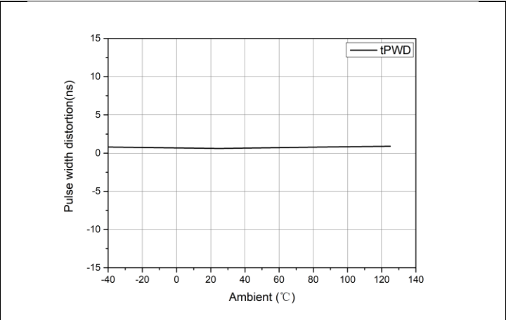
图 7-8 脉宽失真与温度关系
