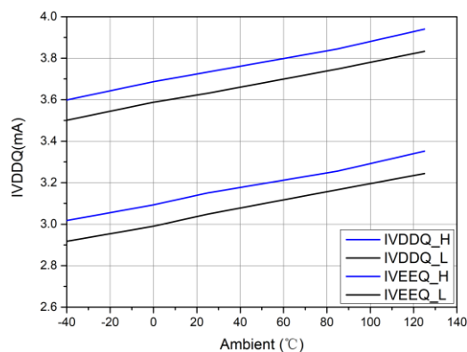
图 7-2 VDD &amp; VEE 静态工作电流与温度关系
