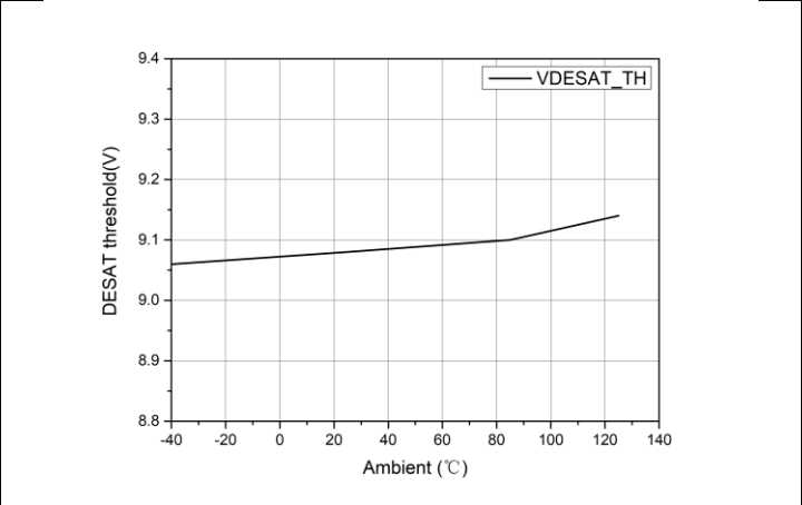
图 7-12 DESAT 电压阈值与温度的关系
