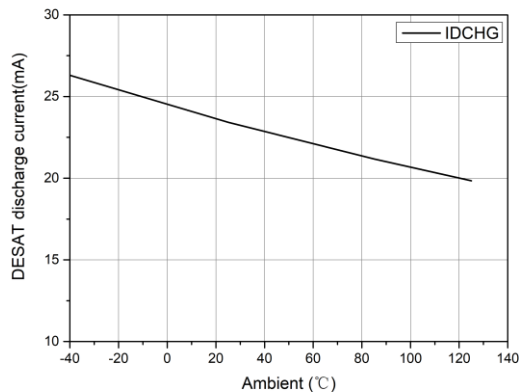
图 7-14 DESAT 放电电流( I_{DCHG} )与温度关系
