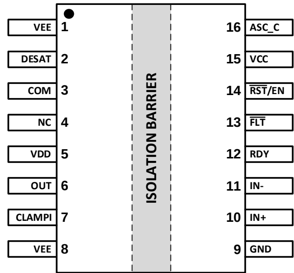
图 6-3 CA-IS3215VNW-Q1 引脚配置
