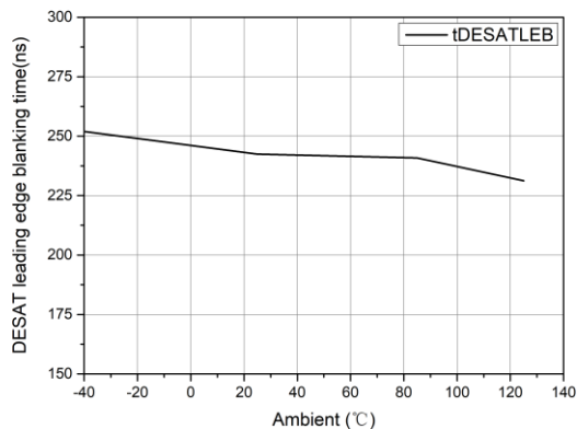
图 7-15 DESAT 消隐时间( t_{DESATLEB} )与温度关系
