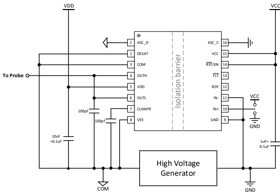
图 8- 16 CMTI 测试方案（CA-IS3215/6xEW）
