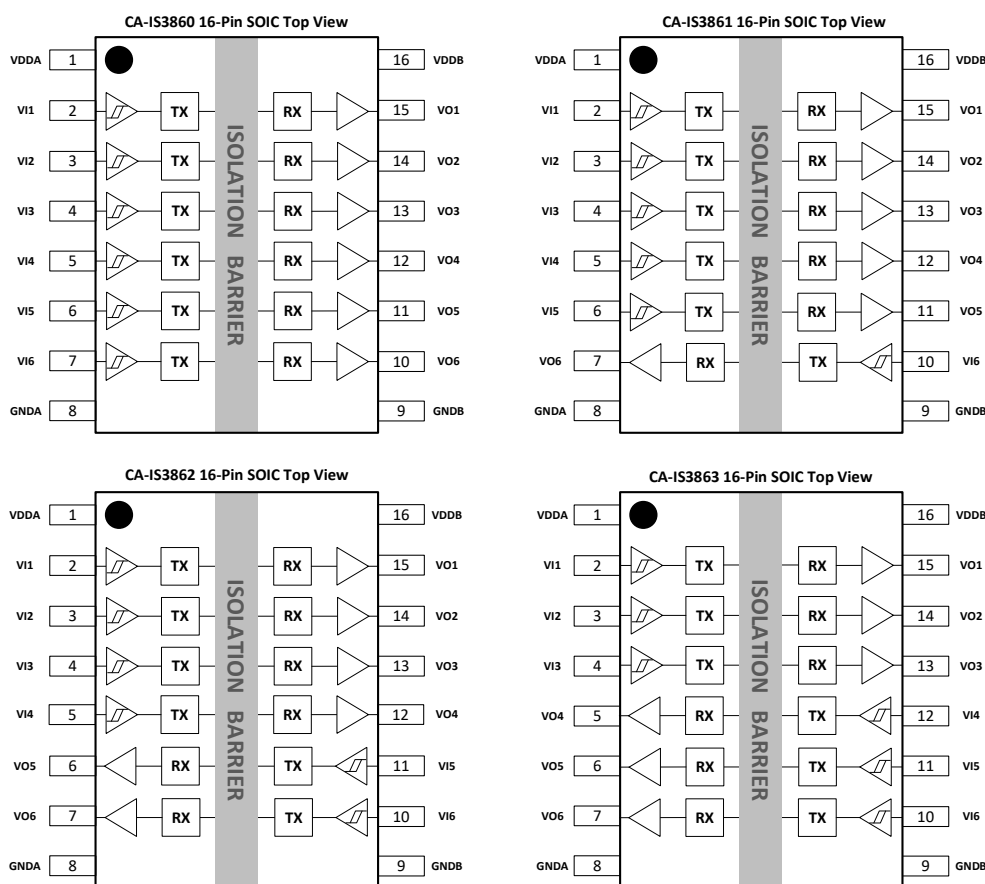
图 6-1 CA-IS386x 顶部视图
