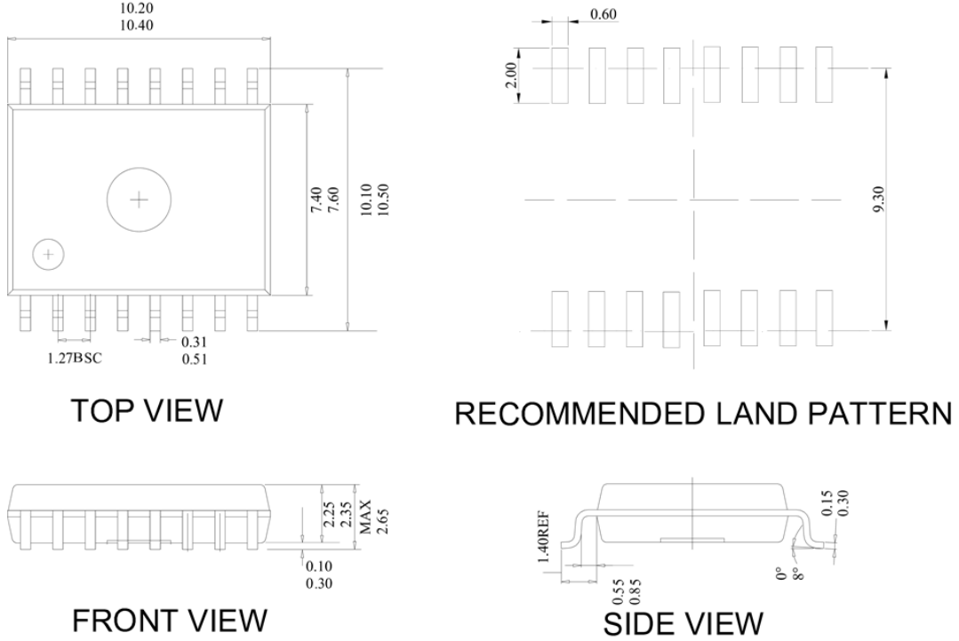
图 11- 1 SOIC16-WB(W)封装尺寸
