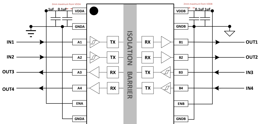
图 10-1 CA-IS3742C 典型应用电路
