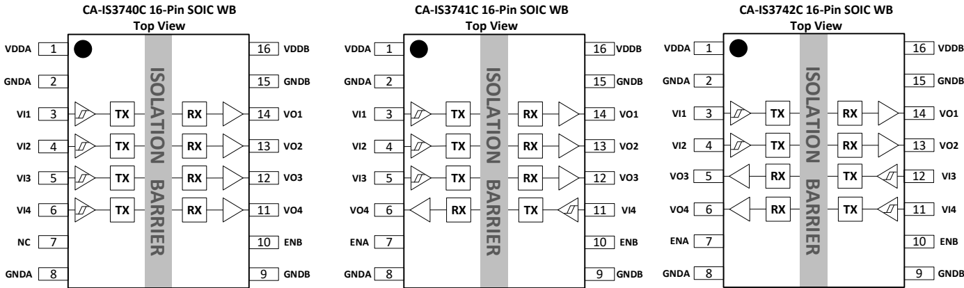
图 6-1 CA-IS374xC 顶部视图
