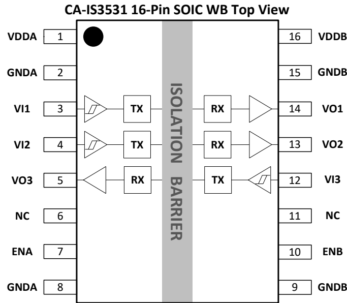
图 7-1 CA-IS3531 顶部视图
