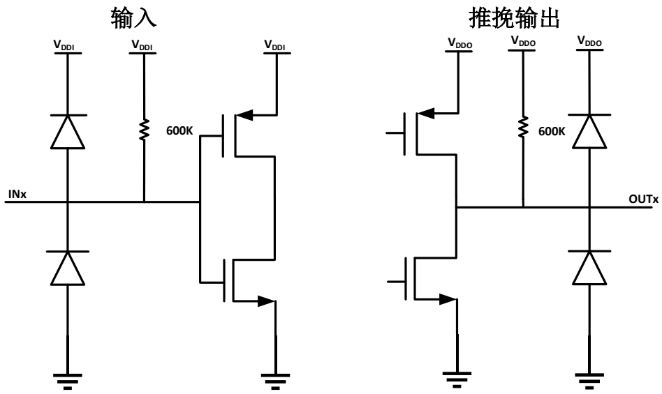
图 11-1 输入输出等效电路
