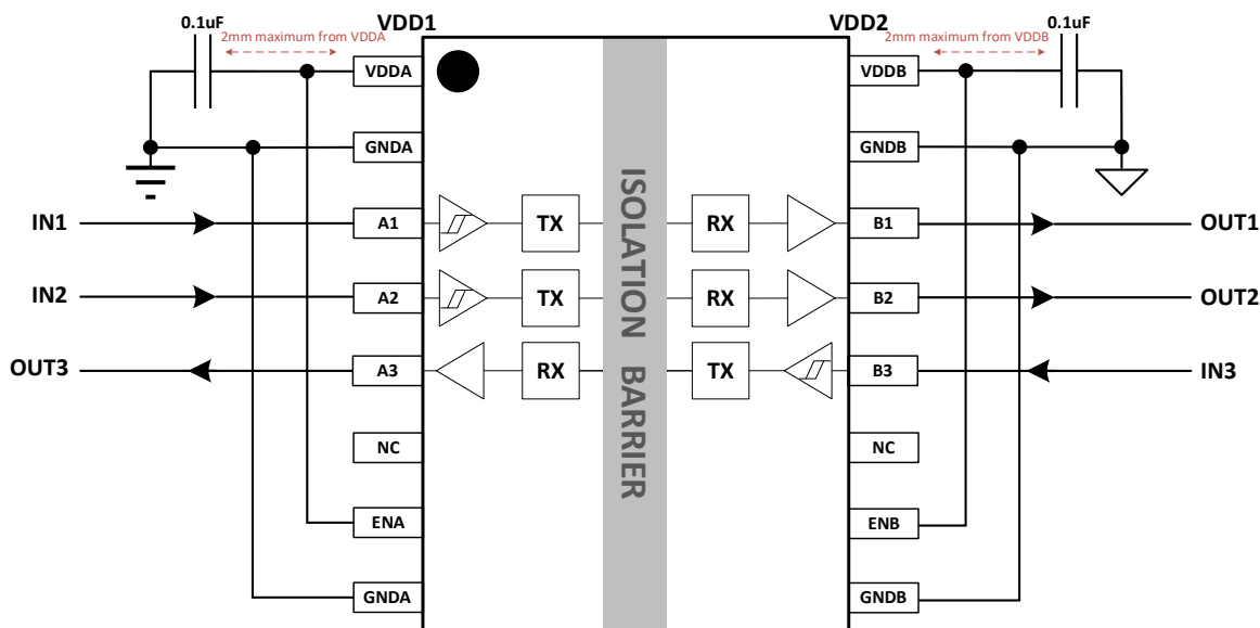
图 12-1 CA-IS3531 典型应用电路
