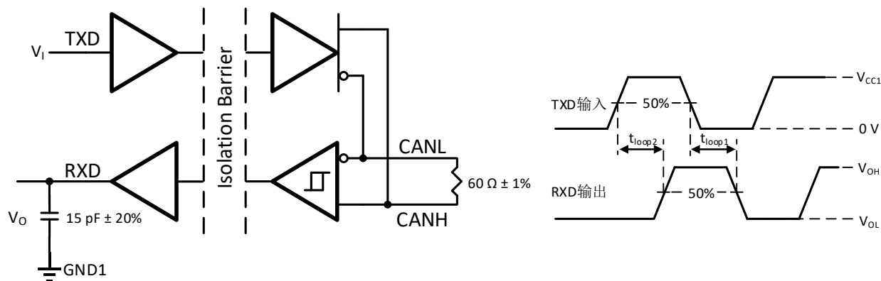
图 8-8 TXD 到 RXD 环路延时
