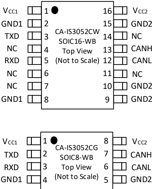
图 6-2 CA-IS3052C 引脚配置
