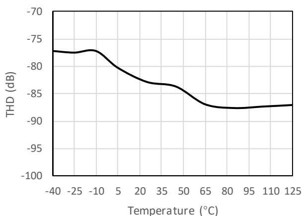
图 7-13 总谐波失真 vs 温度 @ f_{IN} = 10\text{ kHz}
