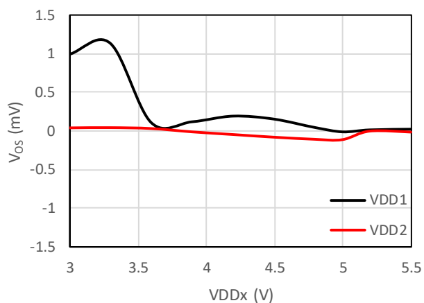
图 7-4 输入失调电压 vs 供电电压
