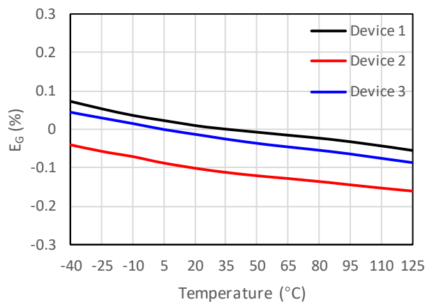
图 7-1 增益误差 vs 温度
