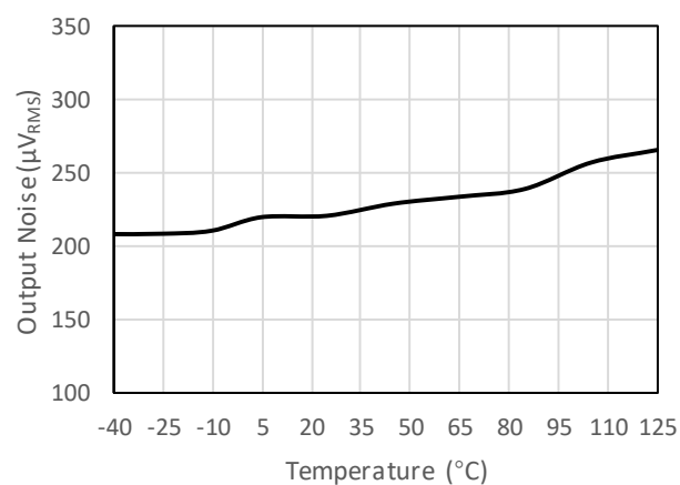
图 7-18 输出噪声 vs 温度 @ V_{IN} = 1\text{ V}
