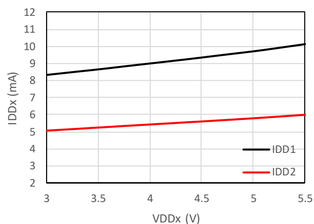
图 7-24 供电电流 vs 供电电压
