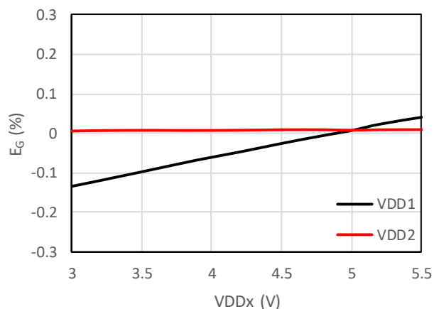
图 7-2 增益误差 vs 供电电压
