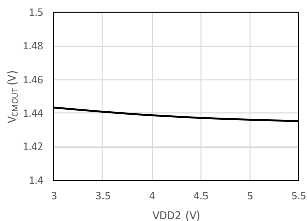
图 7-16 共模输出电压 vs 供电电压
