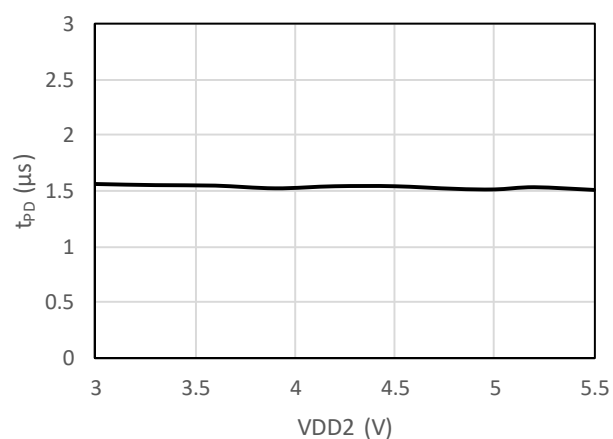
图 7-22 输入输出信号延时 vs 供电电压
