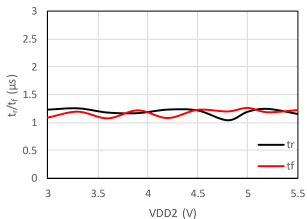
图 7-20 输出上升下降时间 vs 供电电压
