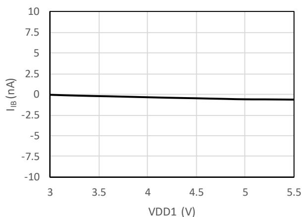
图 7-6 输入电流 vs 供电电压 @ VIN 引脚
