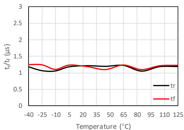
图 7-19 输出上升下降时间 vs 温度
