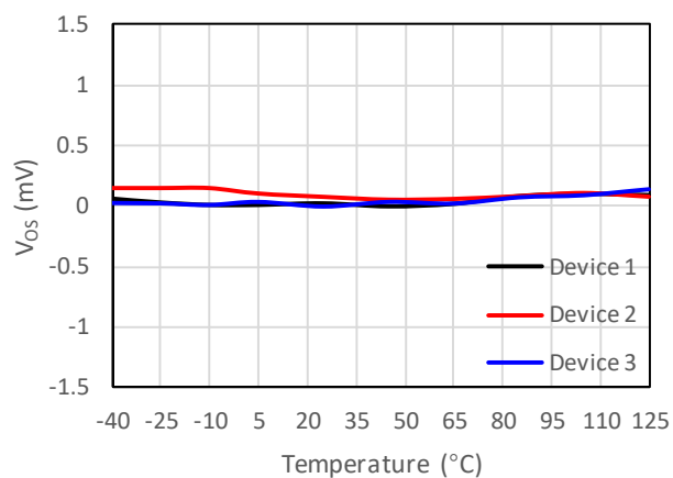
图 7-3 输入失调电压 vs 温度
