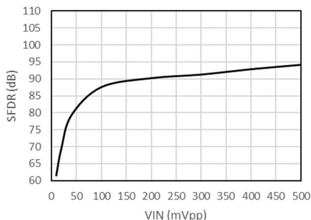
图 7-22 无杂散动态范围 vs 输入
