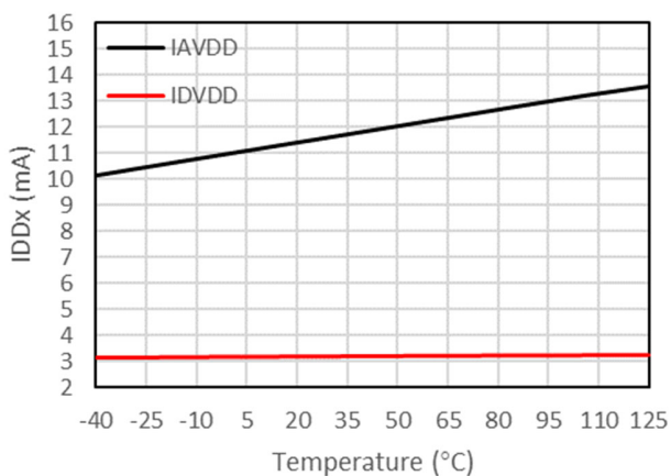
图 7-23 供电电流 vs 温度
