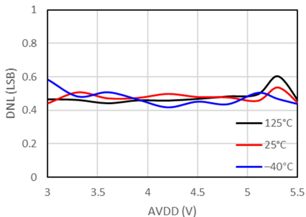
图 7-26 微分非线性 vs 高边供电电压
