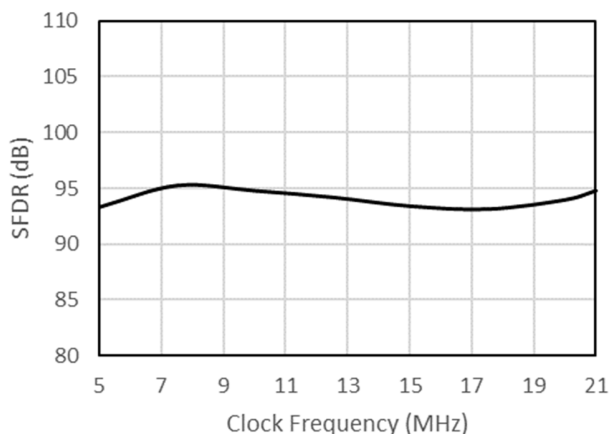
图 7-21 无杂散动态范围 vs 时钟频率
