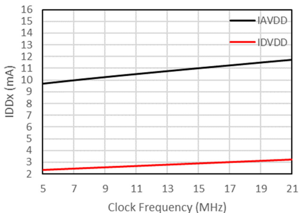
图 7-25 供电电流 vs 时钟频率
