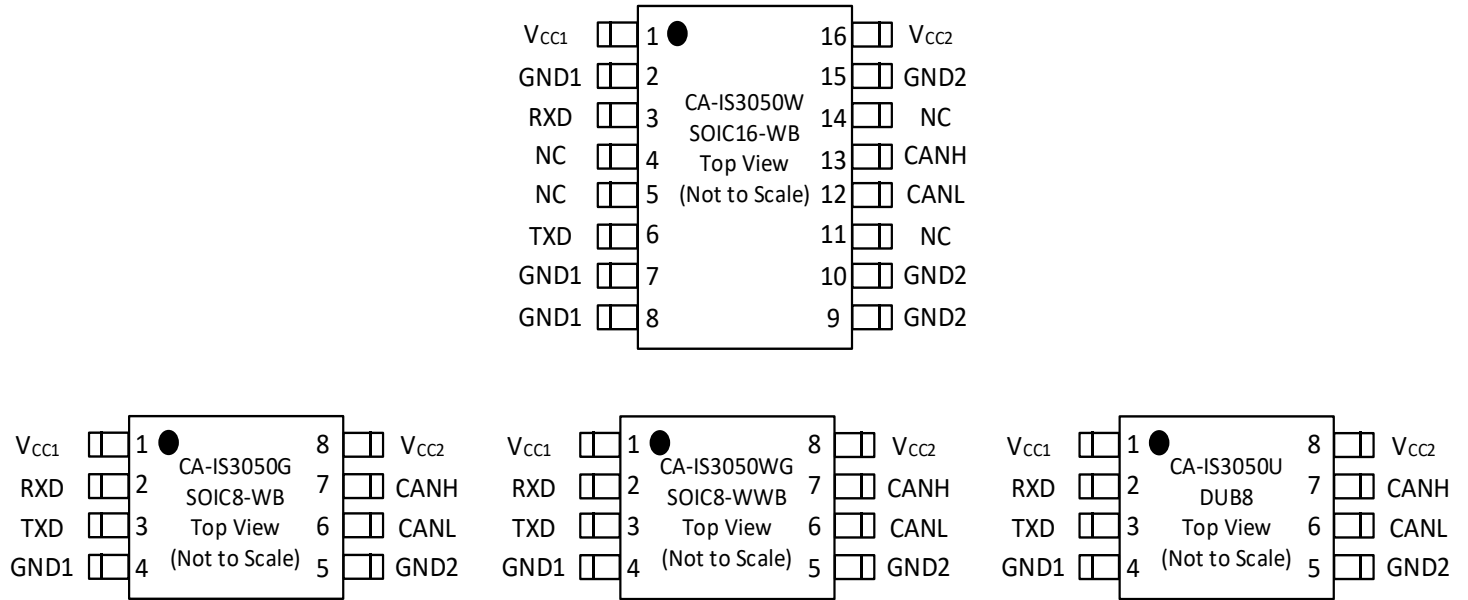
图 6-1 CA-IS3050 引脚配置
