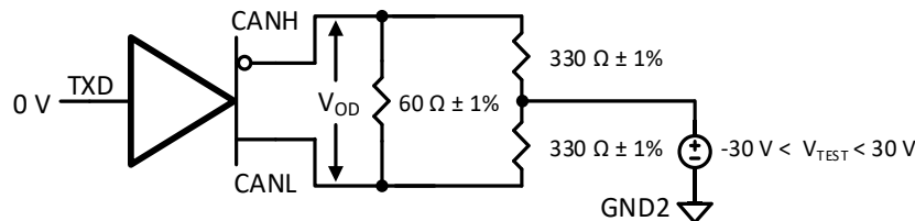
图 8-3 驱动器 V_{OD} 电压测试电路(带共模负载)
