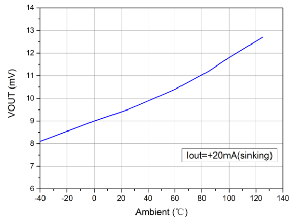
图 7-8 VOL VS. 温度 (20mA Load)
